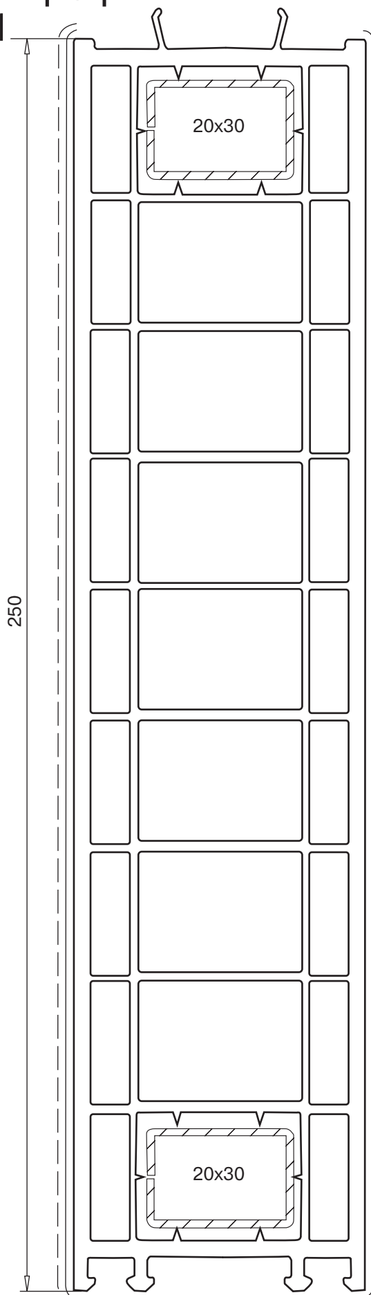
расширитель 250 мм арт. № 114.005 усилитель арт. № 113.019
