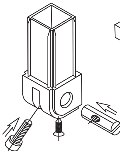
соединитель с изменяемым углом в наборе арт. № 141.313
