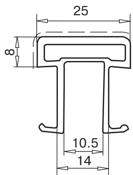
арт. № 116.029
