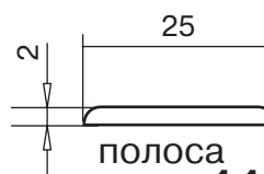
полоса арт. № 117.853
