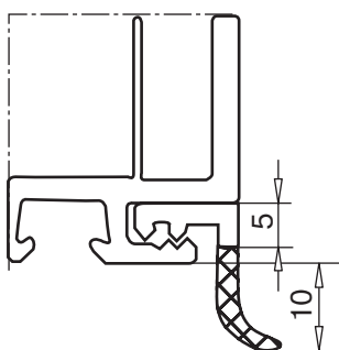
профиль для присоединения к стене арт. № 109.234
