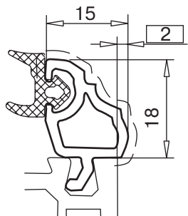
штапик арт. № 107.595
