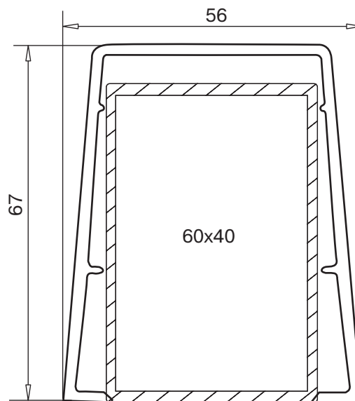
внешний усилитель 56x67 мм арт. № 114.019 усилитель арт. № 113.011.2 I_x=10,23 \text{ см}^4 , I_y=19,31 \text{ см}^4 усилитель арт. № 113.011.3 I_x=14,32 \text{ см}^4 , I_y=27,39 \text{ см}^4
