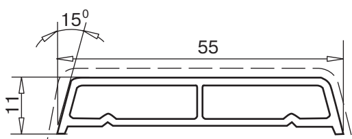
перекладина 11x55 мм арт. № 109.277 крепление на силиконе
