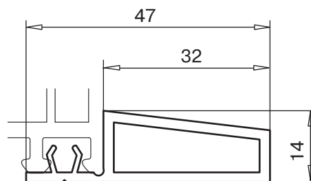
маскирующий профиль арт. № 109.231
