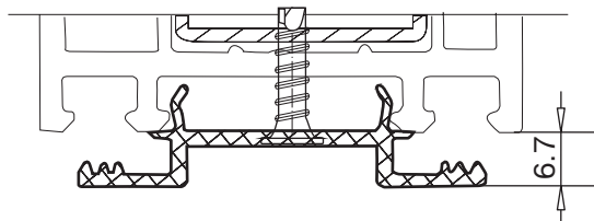
адаптор из алюминия арт. № 109.338 цвет: алюминиевый
