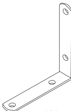
соединительный уголок арт. № 141.400.7 83,5/83,5/20мм
