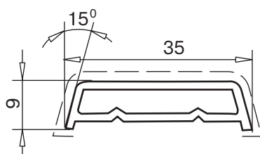
перекладина 9x35 мм арт. № 109.276 крепление на силиконе
