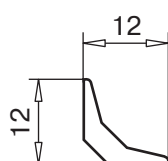
закрывающая планка арт. № 117.855
