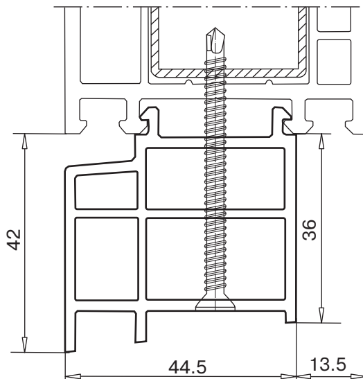
профиль для присоединения отлива арт. № 110.026
