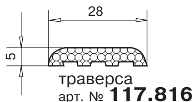
траверса арт. № 117.815
