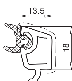
штапик арт. № 107.582
