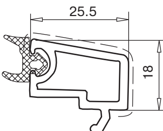
штапик арт. № 107.568
