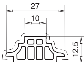
перекладка фигурная арт. № 109.412.2 с клейкой лентой
