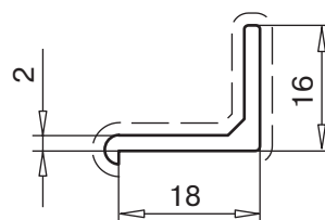
упорная планка для раздвижной складывающейся двери арт. № 109.274
