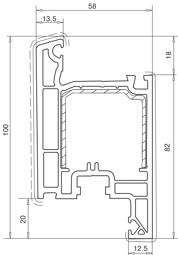
створка 100мм нсв открывается внутрь арт. № 103.198 усилитель арт. № 113.147.2
