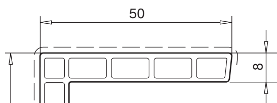
полый уголок арт. № 111.032
