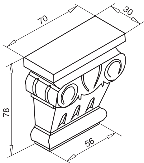
декоративная капитель арт. № 146.161 цвет: белый
