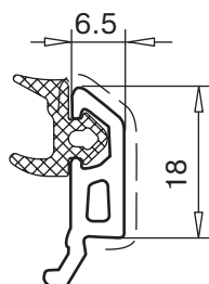
штапик арт. № 107.528
