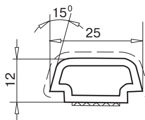
перекладина 12x25 мм арт. № 109.389.2 с клейкой лентой
