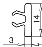
заглушка из ПВХ арт. № 109.037 для порога 104.037 цвет: белый, коричневый
