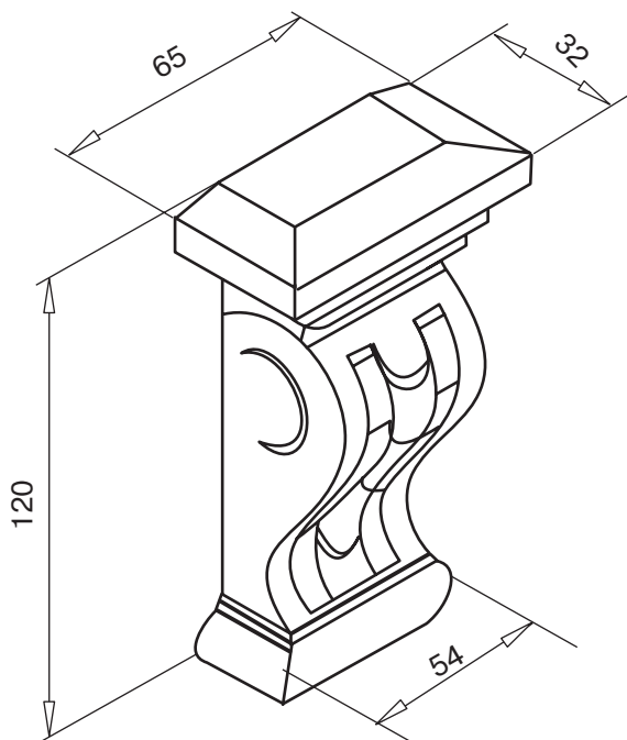
декоративная капитель арт. № 146.162 цвет: белый
