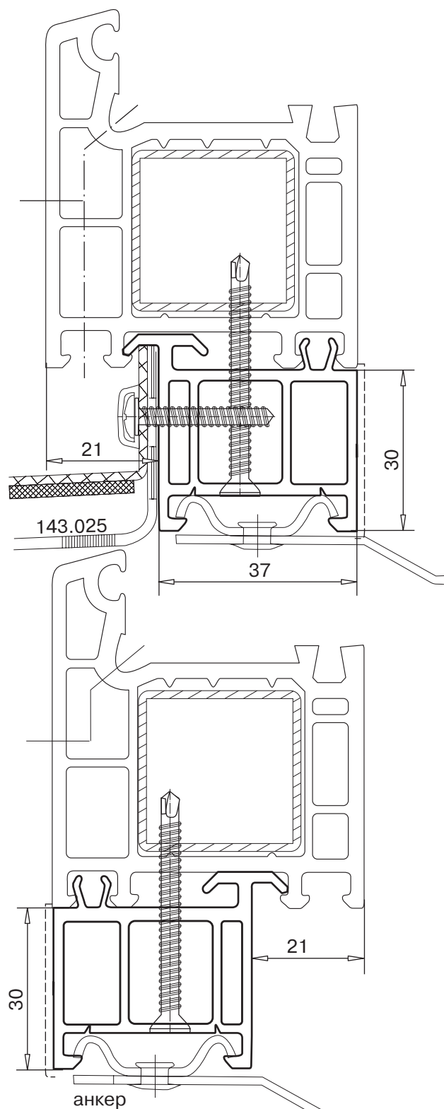
профиль для присоединения балконной двери 30мм арт. № 109.304
