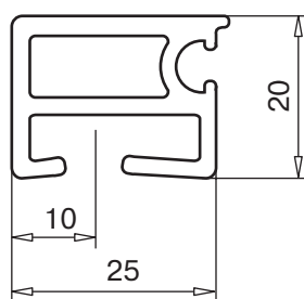
маскирующий профиль арт. № 109.020
