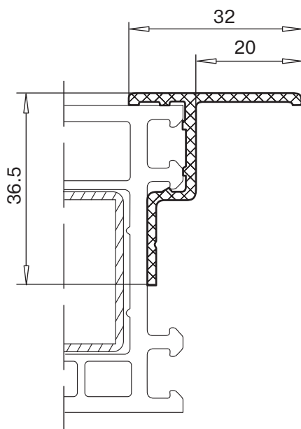
соединитель из алюминия арт. № 116.022 цвет: белый
