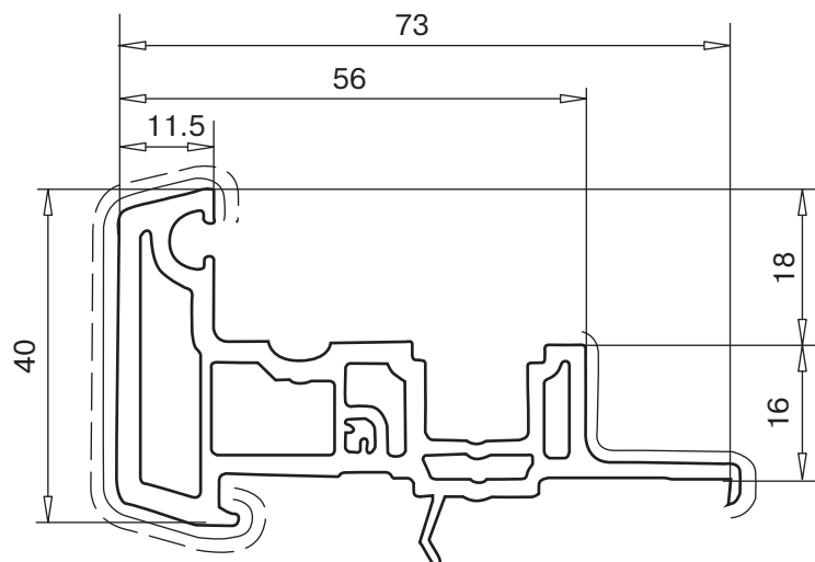
штульп 40мм арт. № 102.197
