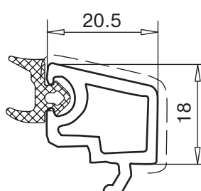
штапик арт. № 107.567
