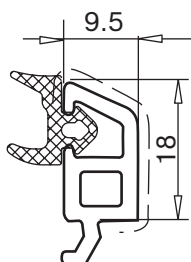
штапик арт. № 107.517
