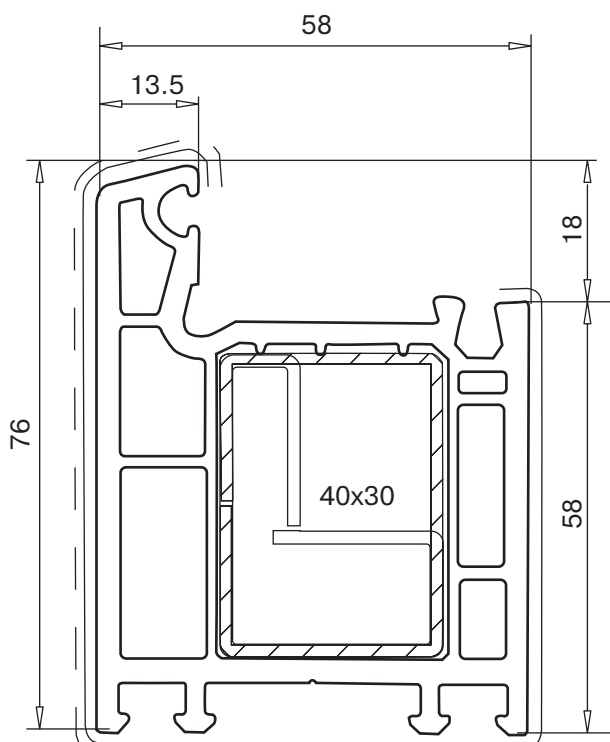
рама 76 мм арт. № 101.111 усилитель арт. № 113.001 усилитель для входной двери арт. № 113.009
