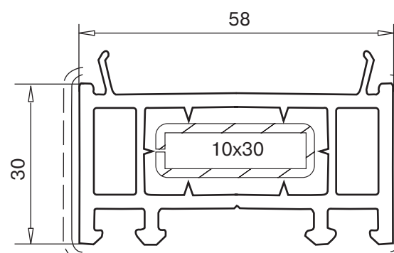
расширитель 30 мм арт. № 114.012 усилитель арт. № 113.020
