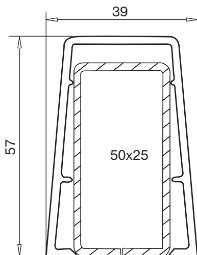
внешний усилитель 39x57 мм арт. № 114.018 усилитель арт. № 113.161.3 I_x=3,99 \text{ см}^4 , I_y=12,55 \text{ см}^4
