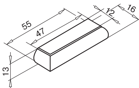
декоративная капитель- соединитель арт. № 146.163 цвет: белый
