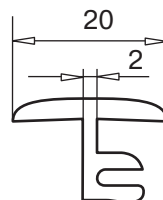
соединитель мини выступс одной стороны арт. № 116.005.2
