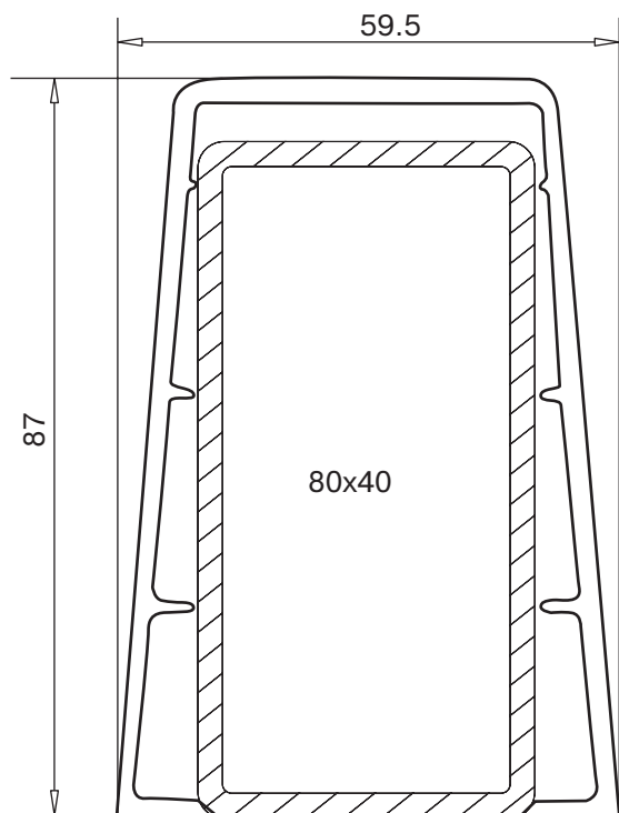
внешний усилитель 59,5x87 мм арт. № 114.020 усилитель арт. № 113.015.3 I_x=18,50 \text{ см}^4 , I_y=55,50 \text{ см}^4
