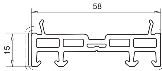
расширитель 15 мм арт. № 114.024
