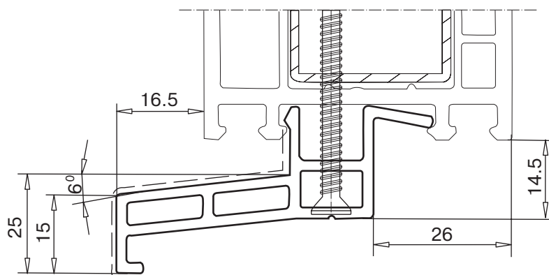
профиль для присоединения отлива арт. № 110.028
