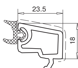
штапик арт. № 107.583
