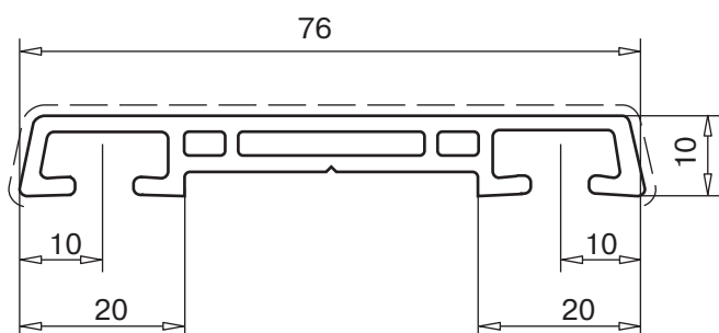
облицовочный профиль арт. № 109.208
