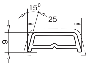
перекладина 9x25 мм арт. № 109.275 крепление на силиконе
