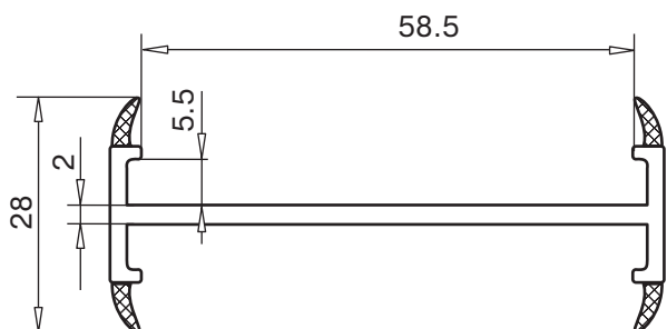
соединительный профиль арт. № 116.013 с белыми уплотнениями
