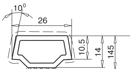
перекладка 14x26 мм арт. № 109.105.2 с клейкой лентой
