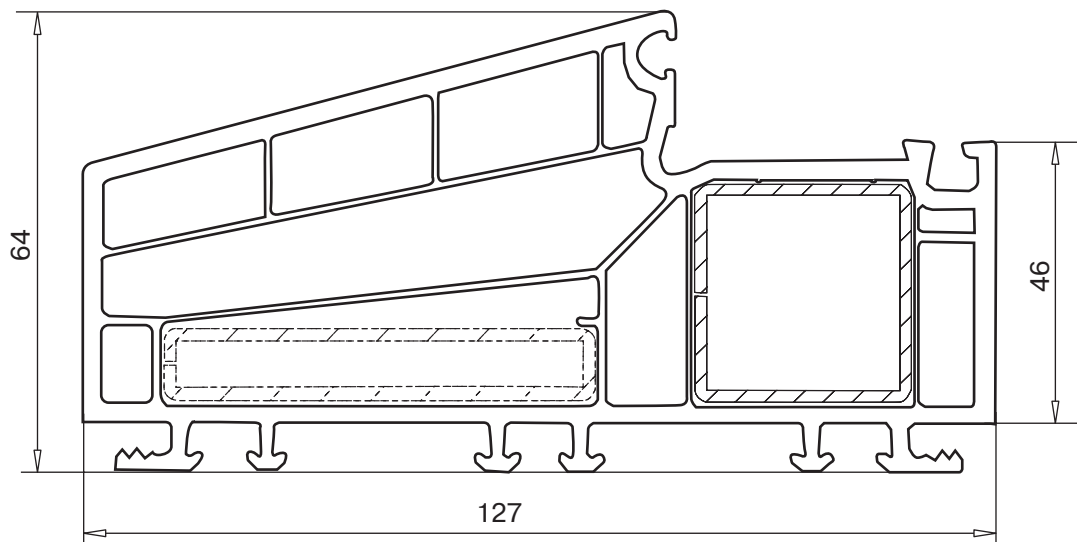
рама 64 мм арт. № 101.151 в белом исполнении
