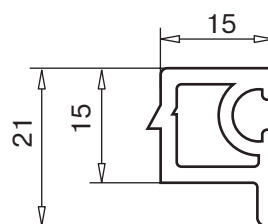
заполняющий профиль арт. № 109.343
