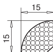
четвертушка арт. № 117.817
