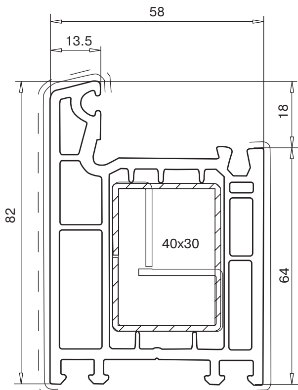
рама 82 мм арт. № 101.085 усилитель арт. № 113.001 усилитель для входной двери арт. № 113.009
