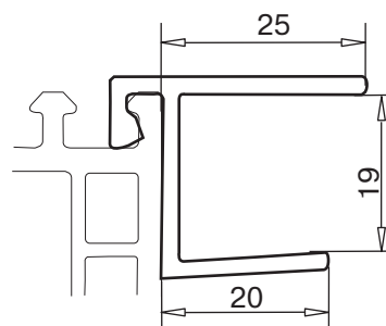
профиль с пазом арт. № 109.342
