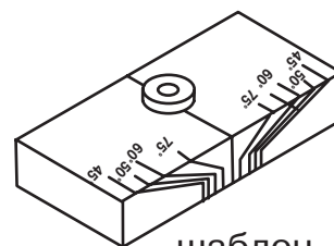
шаблон арт. № 146.011.9 для соединения переклад. 141.313
