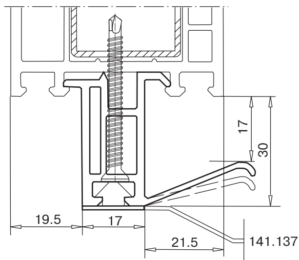
профиль для присоединения подоконника арт. № 110.054 для подоконника 17-22 мм анкер с захватом 141.137
