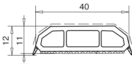
перекладина 12x40 мм арт. № 109.504.2 с клейкой лентой
