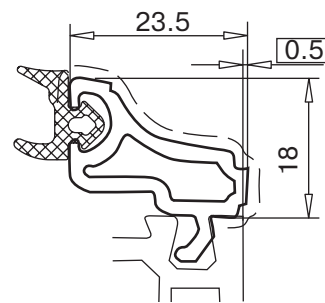
штапик арт. № 107.555
