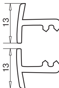
соединительный профиль арт. № 116.018.2
