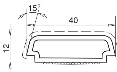
перекладина 12x40 мм арт. № 109.388.2 с клейкой лентой
