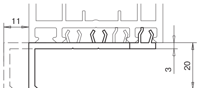
4 соединительный профиль арт. № 109.071
