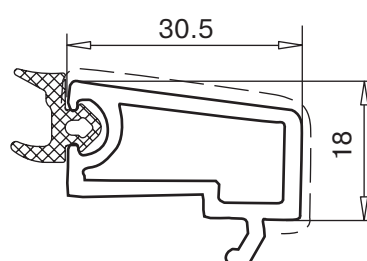
штапик арт. № 107.569
