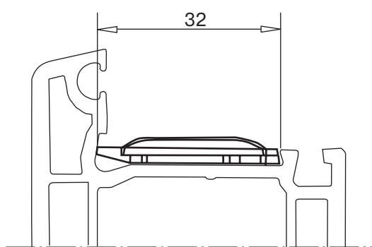
фальцевый вкладыш НСВ арт. № 109.293 цвет: зеленый
