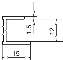
стыкующий профиль арт. № 117.849
