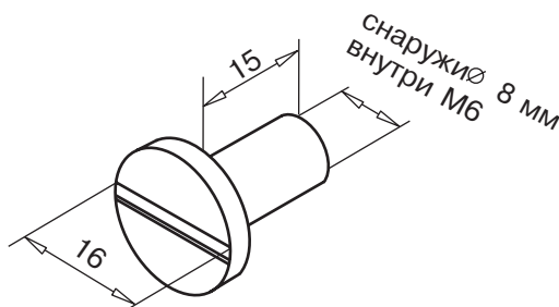
гильза для SL AD арт. № 141.124.2 никелированная латунь
