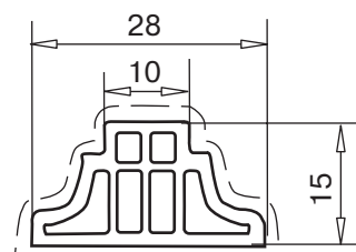
перекладка фигурная арт. № 109.114
