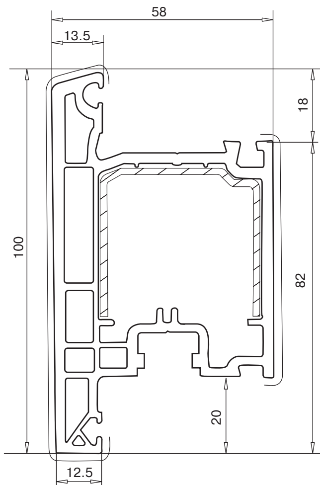
створка 100мм нсв открывается наружу арт. № 103.219 усилитель арт. № 113.147.2
