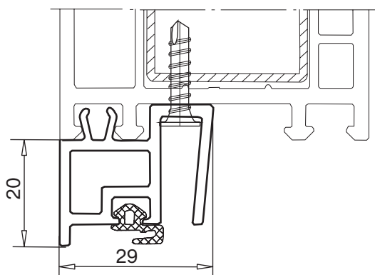
профиль для присоединения отлива арт. № 110.023 уплотнение арт. № 112.072
