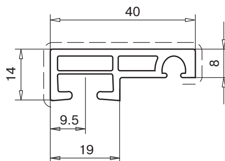
облицовочный профиль арт. № 109.104
