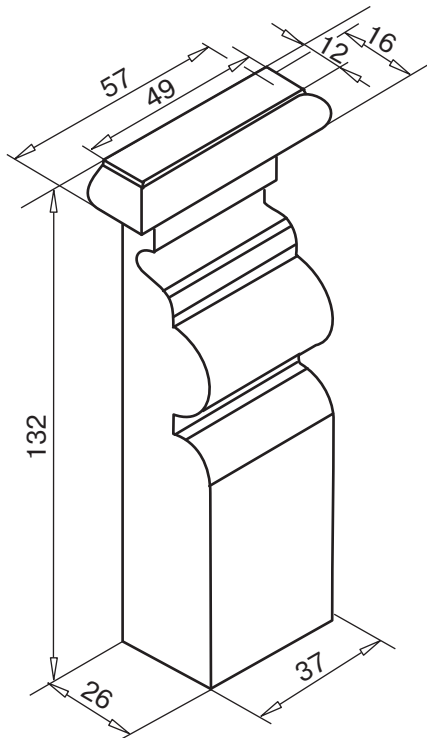
декоративная капитель арт. № 146.164 цвет: белый
