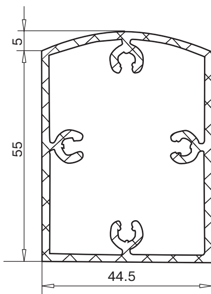
порог для входной двери арт. № 104.009 цвет: алюмин., E6/EV1, Euras 15
