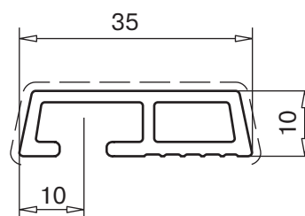
облицовочный профиль арт. № 109.211
