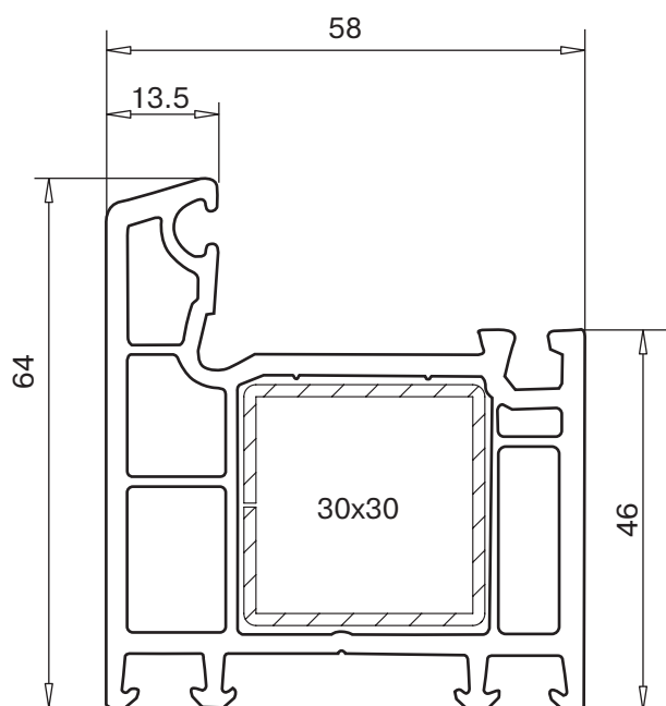
арт. № 101.213 усилитель арт. № 113.025
