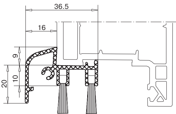
алюминиевая защитная планка арт. № 104.116 цвет: белый, коричневый
