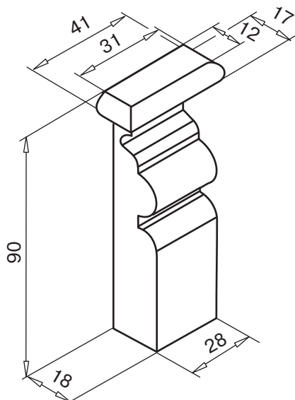
декоративная капитель арт. № 146.174 цвет: белый
