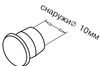
заглушка \varnothing 10 мм арт. № 141.154 цвет: белый
