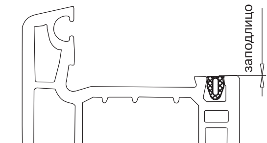
заполняющее уплотнение арт. № 112.380 цвет белый, охра, черный
