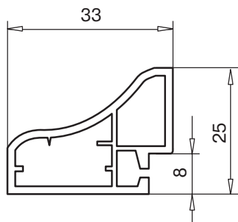
профиль для отделки откоса арт. № 109.106
