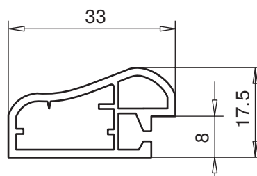
профиль для отделки откоса арт. № 109.107
