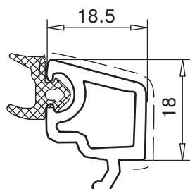
штапик арт. № 107.591
