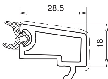
штапик арт. № 107.592
