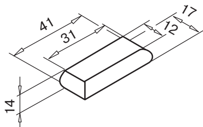
декоративная капитель- соединитель арт. № 146.173 цвет: белый
