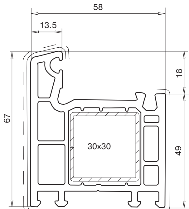
рама 67 мм арт. № 101.086 усилитель арт. № 113.025
