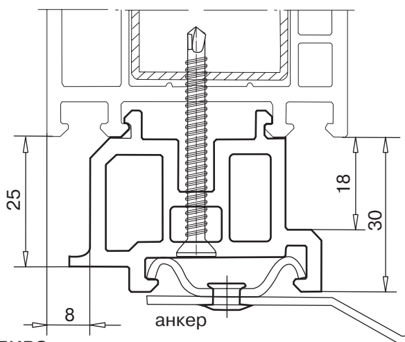
профиль для присоединения отлива арт. № 110.005
