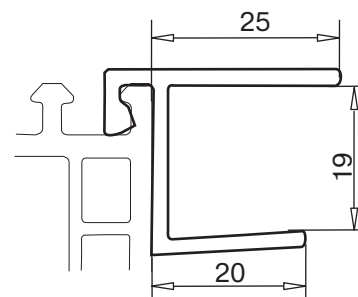
профиль с пазом арт. № 109.342
