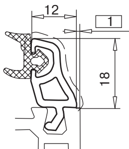
штапик арт. № 107.580
