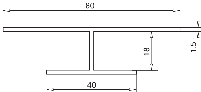
соединительный профиль арт. № 117.831
