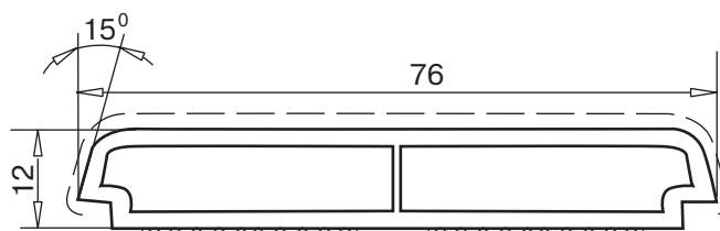
перекладина 12x76 мм арт. № 109.387.2 с клейкой лентой
