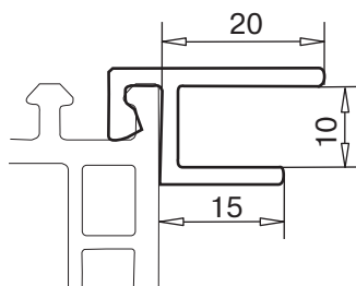
П-образный профиль арт. № 109.254
