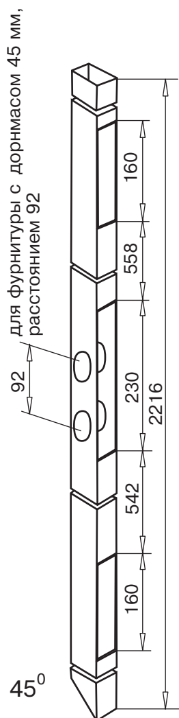
арт. № 113.005.5 60x45x3 мм длина 2216 мм
