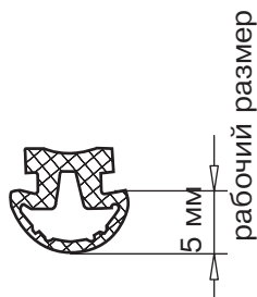
дверное уплотнение арт. № 112.026 цвет: черный
