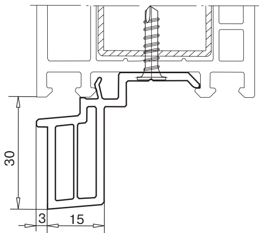
профиль для присоединения отлива арт. № 110.038
