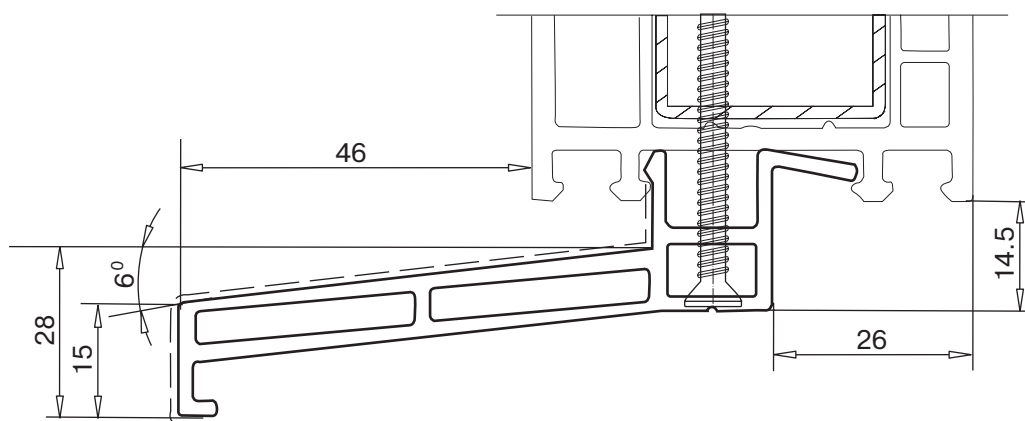
профиль для присоединения отлива арт. № 110.029
