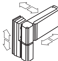
арт. № 140.318 петля VEKA для входной двери из двух частей, для створки весом до 120kg регулируется в 3 плоскостях, установка с обеих сторон цвет: белый / Euras 15 (коричневый) шаблон арт. № 146.011.7
