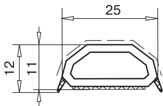
перекладина 12x25 мм арт. № 109.505.2 с клейкой лентой
