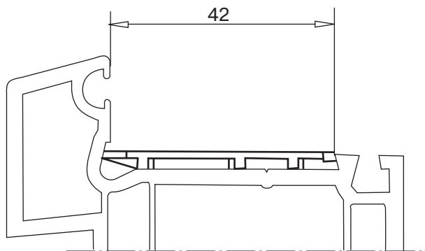
фальцевый вкладыш СВ арт. № 109.294 цвет: желтый
