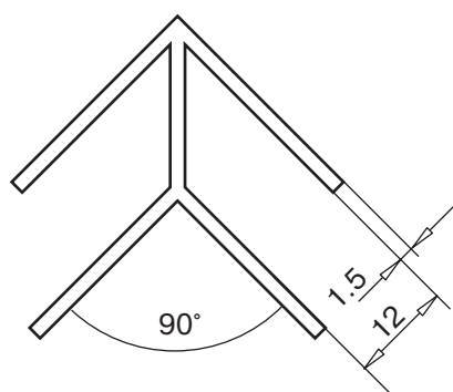
уголок арт. № 117.852
