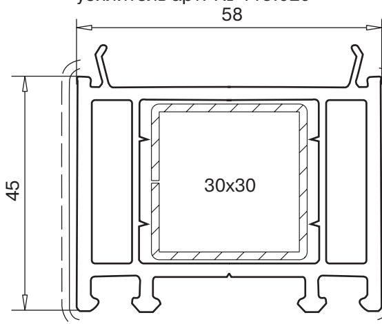
расширитель 30 мм арт. № 114.012 усилитель арт. № 113.020
