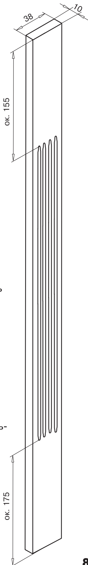
декоративная планка арт. № 146.165 длина 590мм арт. № 146.166 длина 800мм цвет: белый
