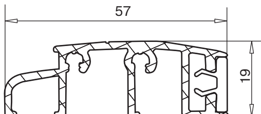
порог для входной двери арт. № 104.037 цвет: алюминий, белый, коричневый
