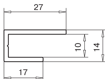
П-образный профиль арт. № 109.254
