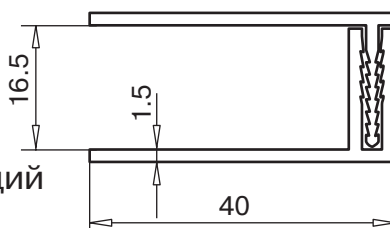
уголок арт. № 117.836
