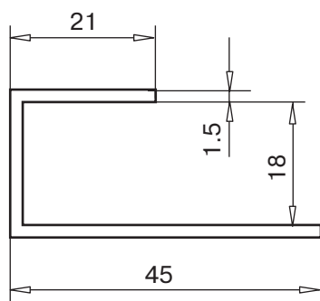
П-образный профиль арт. № 117.833
