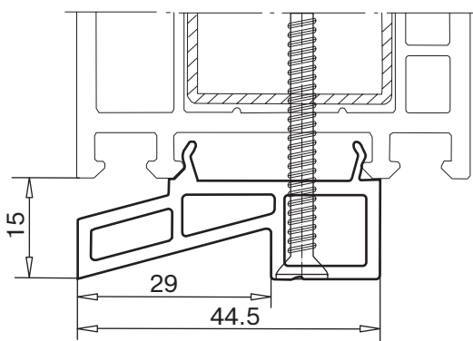
профиль для присоединения отлива арт. № 110.019
